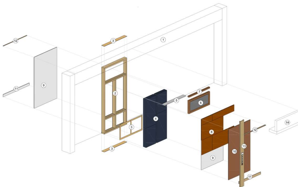
Composition de la cloison couloir/salle isolée coupe feu
