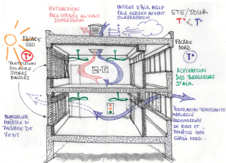
Coupe - fonctionnement bioclimatique après travaux © Passerelle Transition Ecologique
