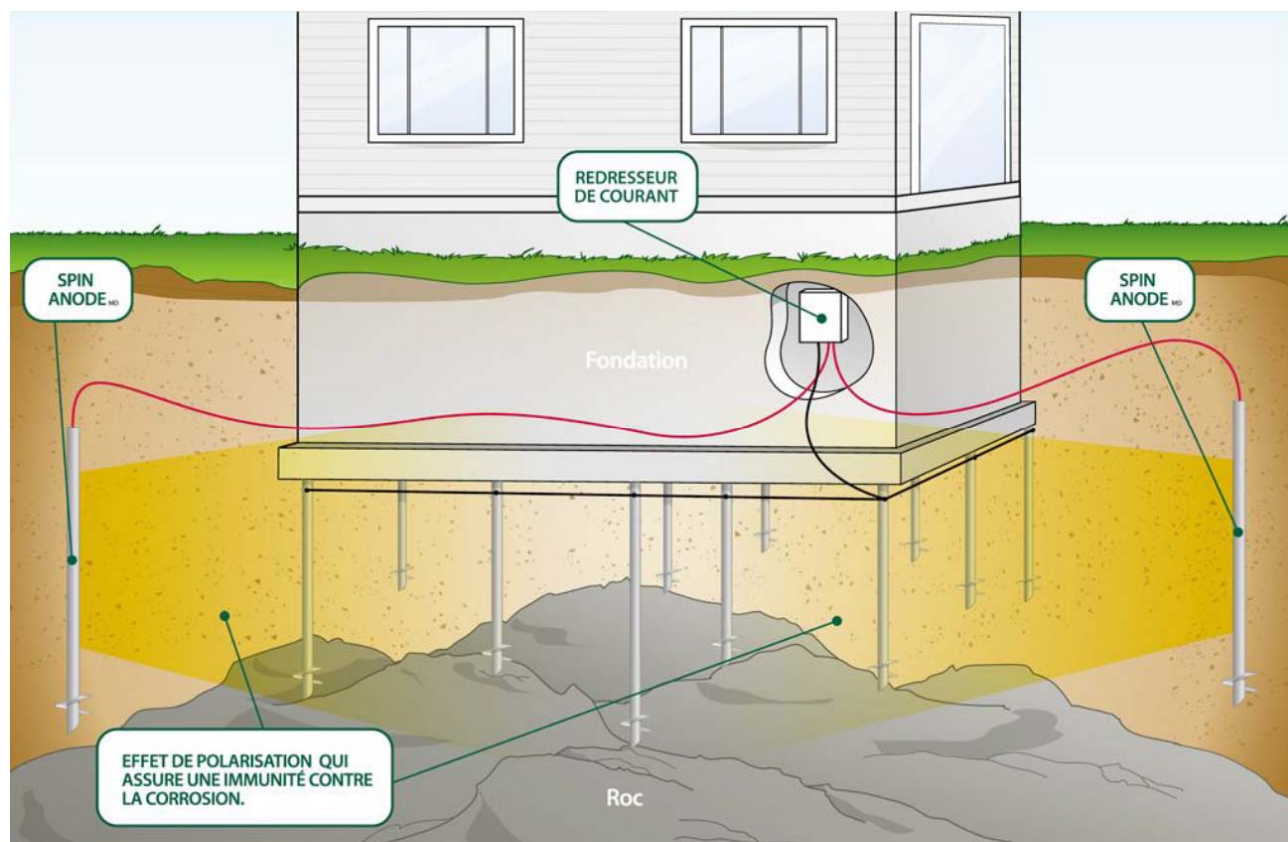
Figure 9 - Fonctionnement de la protection cathodique
