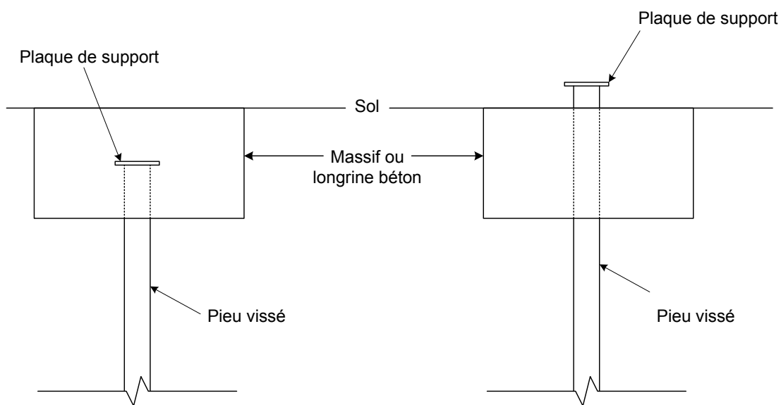
Figure 7 - Principe d'assemblage : cas massif béton
