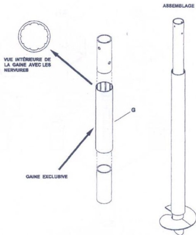
Figure 2 - Assemblage des éléments constituant les TECHNO PIEUX®
