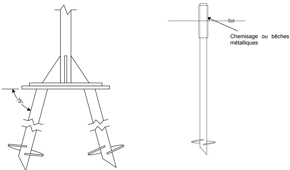
Figure 8 –Dispositions constructives pour la reprise des charges latérales en tête des TECHNO PIEUX® (hors zone sismique pour les pieux obliques)
